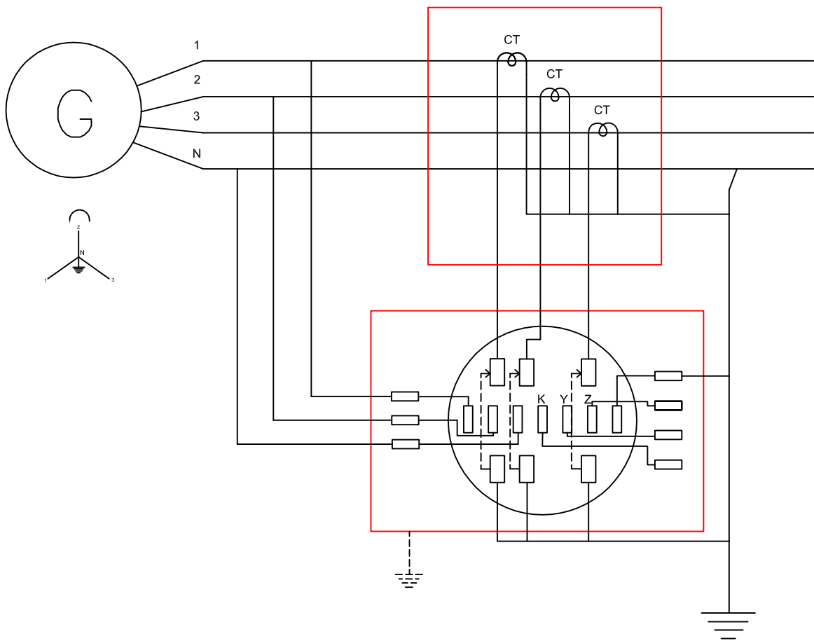
Conexión de medidor 9s, 3 fases, 4 hilos en estrella, 3 CT's y 3 PT's
