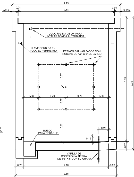
SECCION "B" SIN ESCALA
