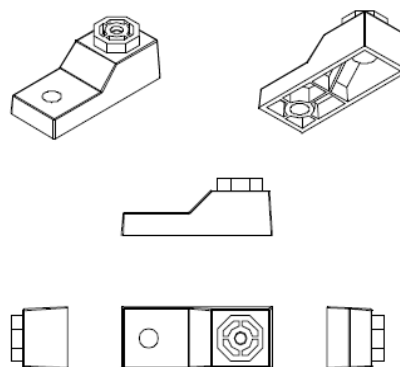
HERRAJE PARA COLOCACIÓN SOBRE MURO ( NO INCLUIDO EN EL SUMINISTRO )
