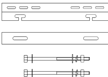
HERRAJE PARA COLOCACIÓN EN POSTE
